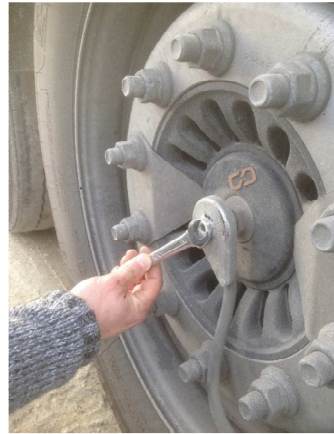
Revisser à l'aide d'une clef de 14 l'enjoliveur
