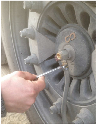
Revisser à l'aide d'une clef de 14 le tuyau
